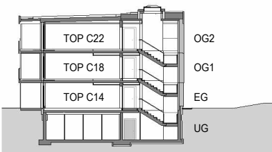
Haus C - Längsschnitt LS
